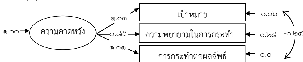
ภาพที่ ๓.๔ องค์ประกอบยืนยันตามโมเดลการวัดองค์ประกอบความคาดหวัง
